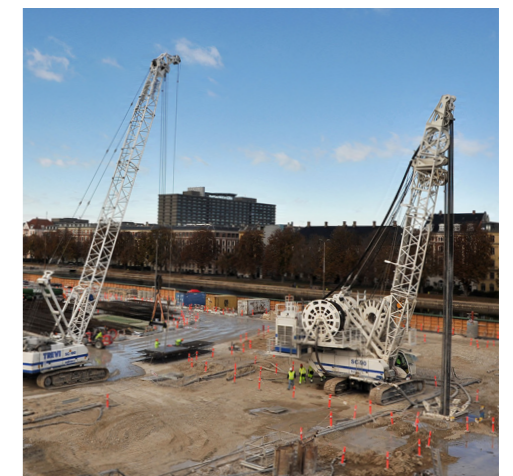
Fondazioni Metro Copenhagen - Danimarca
